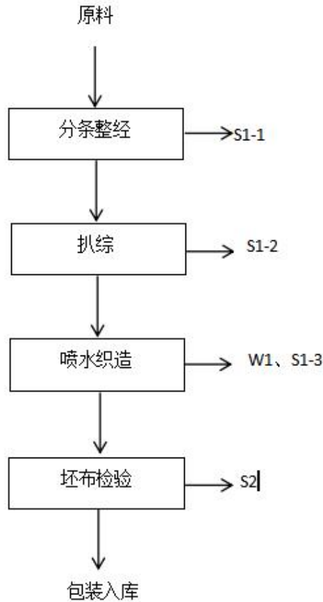
图2-4现有项目生产及产污环节示意图
