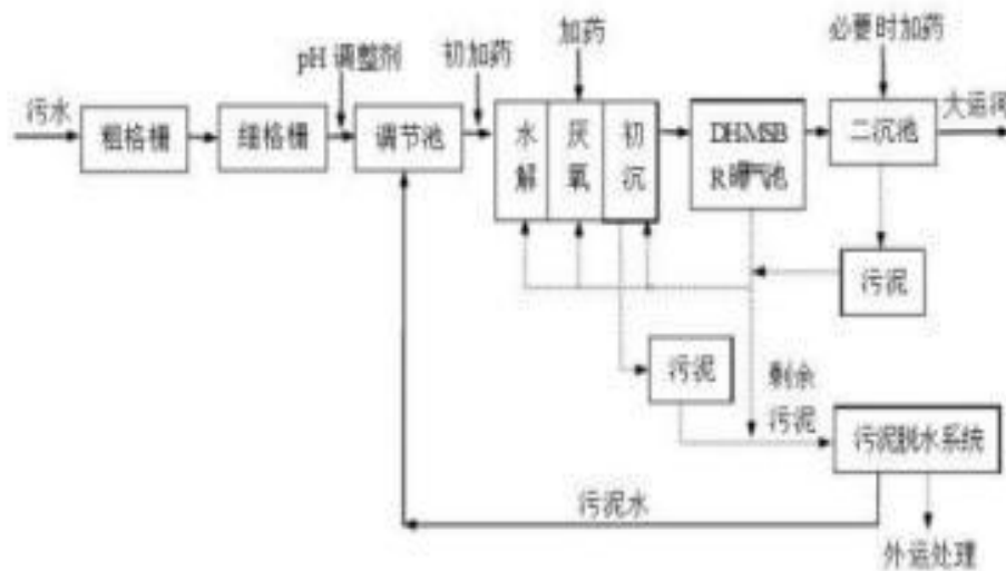
图4-1污水处理厂处理工艺图
