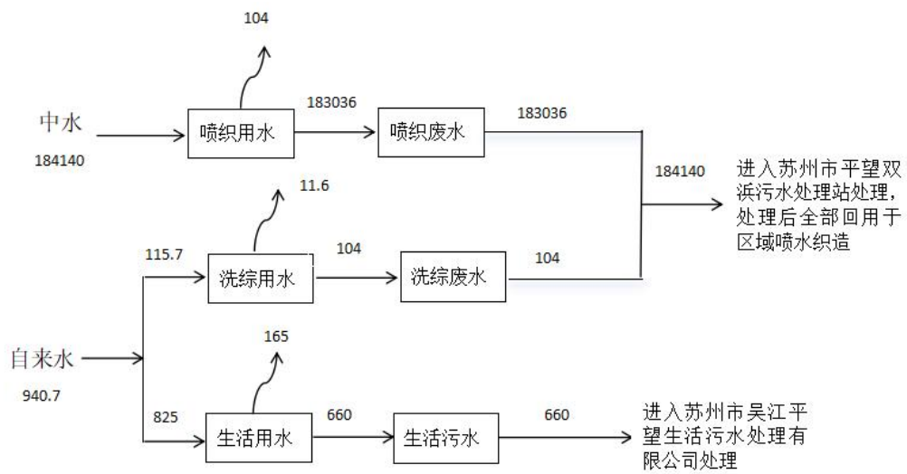
图2-1 项目改造前水平衡图t/a
