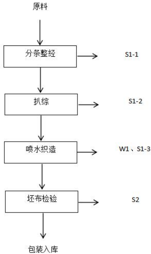
图2-3 生产工艺流程及产污环节示意图
