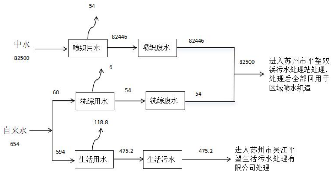
图2-2 项目改造后水平衡图t/a
