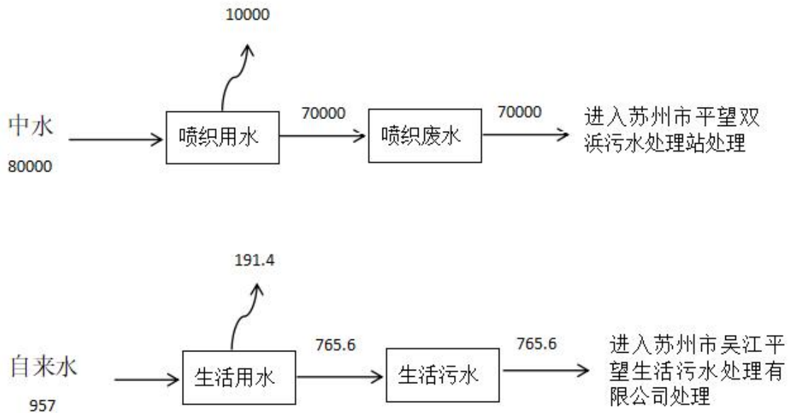
图2-1 项目改造前水平衡图t/a
