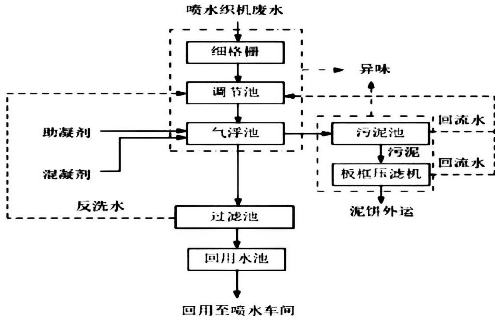
图4-2苏州市双浜污水处理站处理工艺流程
