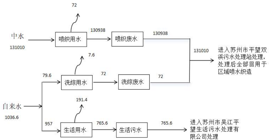
图2-2 本项目改造后水平衡图t/a
